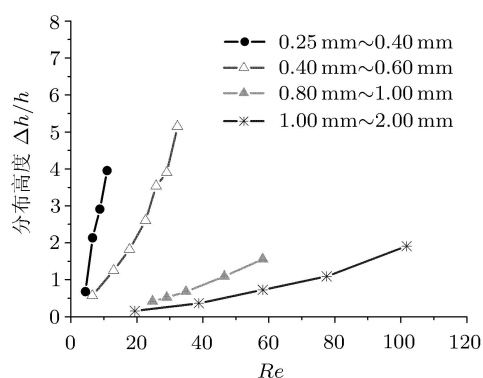
(a) 玻璃珠分布高度随雷诺数的变化
