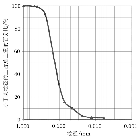
图 2 粉细砂颗粒级配曲线
