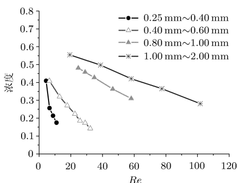
(b) 玻璃珠浓度随雷诺数的变化
