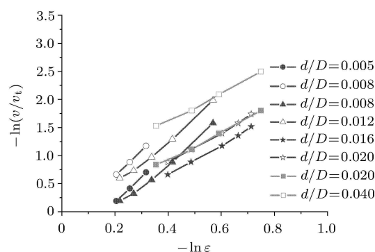
图 4 流速/单颗粒自由沉降速度随水的体积分数的变化
